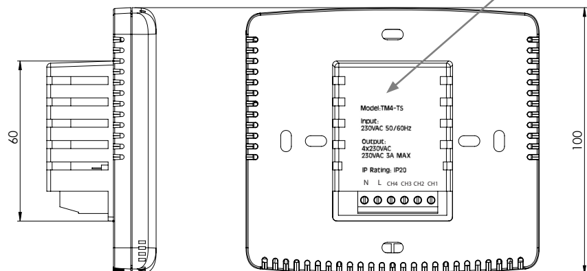
Détails du câblage
