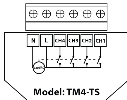
Détails du câblage
