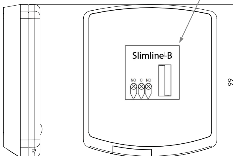
Verdrahtungsdetail
